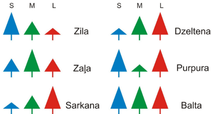
3.zīm. Trīs veidu vāļišu ierosinājuma intensitāte cilvēkam rada attiecīgās krāsas sajūtu. Apzīmējumi: S – īso, M – vidējo un L – garo viļņu jutības vāļītes.
