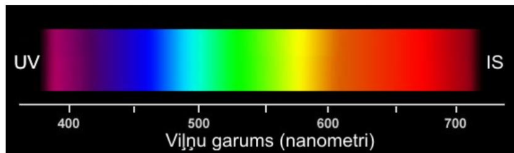
1.zīm. Elektromagnētiskās skalas redzamā gaismas spektra daļa.
