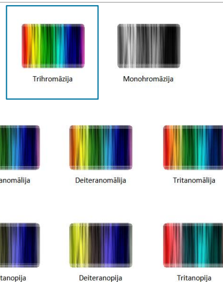
4.zīm. Krāsu uztvere cilvēkam ar neizmainītu krāsu redzi (trihromāzija) un cilvēkam ar krāsu redzes traucējumiem.
